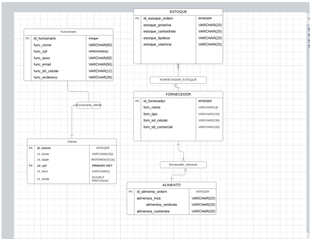
Figura 5 - MFD: Modelo Físico de Dados.
